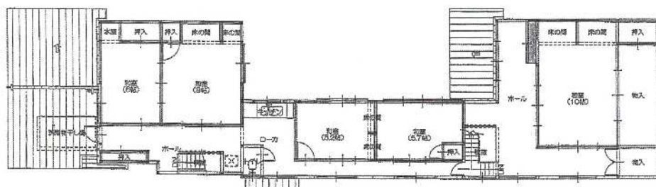
2階 平面図 8:1/100
