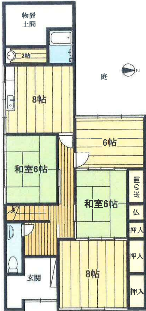
1階平面図
